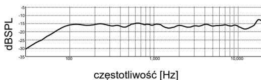
Pasmo przenoszenia
