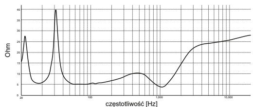
Impedancja
