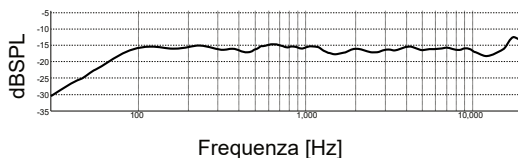
Risposta in frequenza
